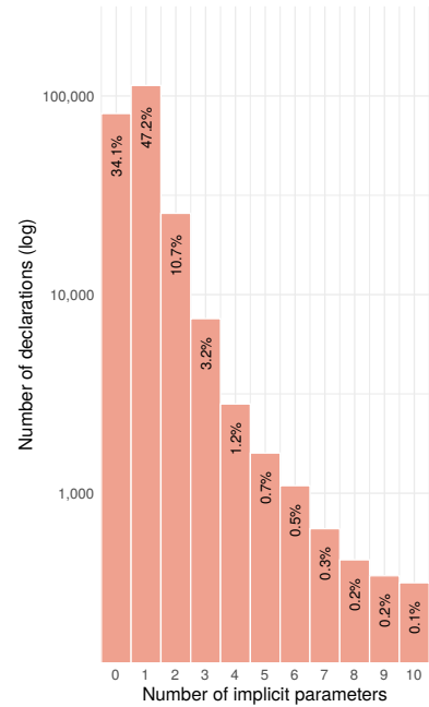
Fig. 10. Implicit parameters
