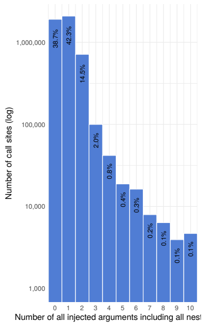
Fig. 9. Injected arguments
